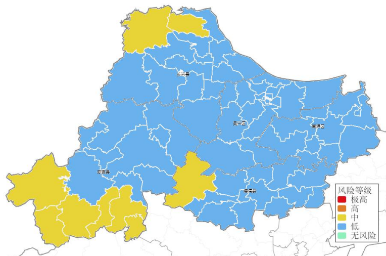
3 月 26 日 20 时至 27 日 20 日强对流致灾风险预警等级图
